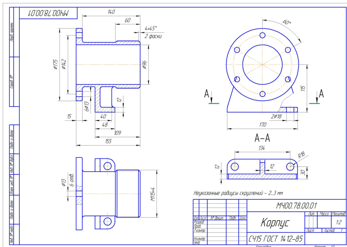
Рис. 11. Графическая работа по разделу «Инженерная графика». Тема «Деталирование чертежа общего вида». (Лист 6-9 – чертежи деталей)
