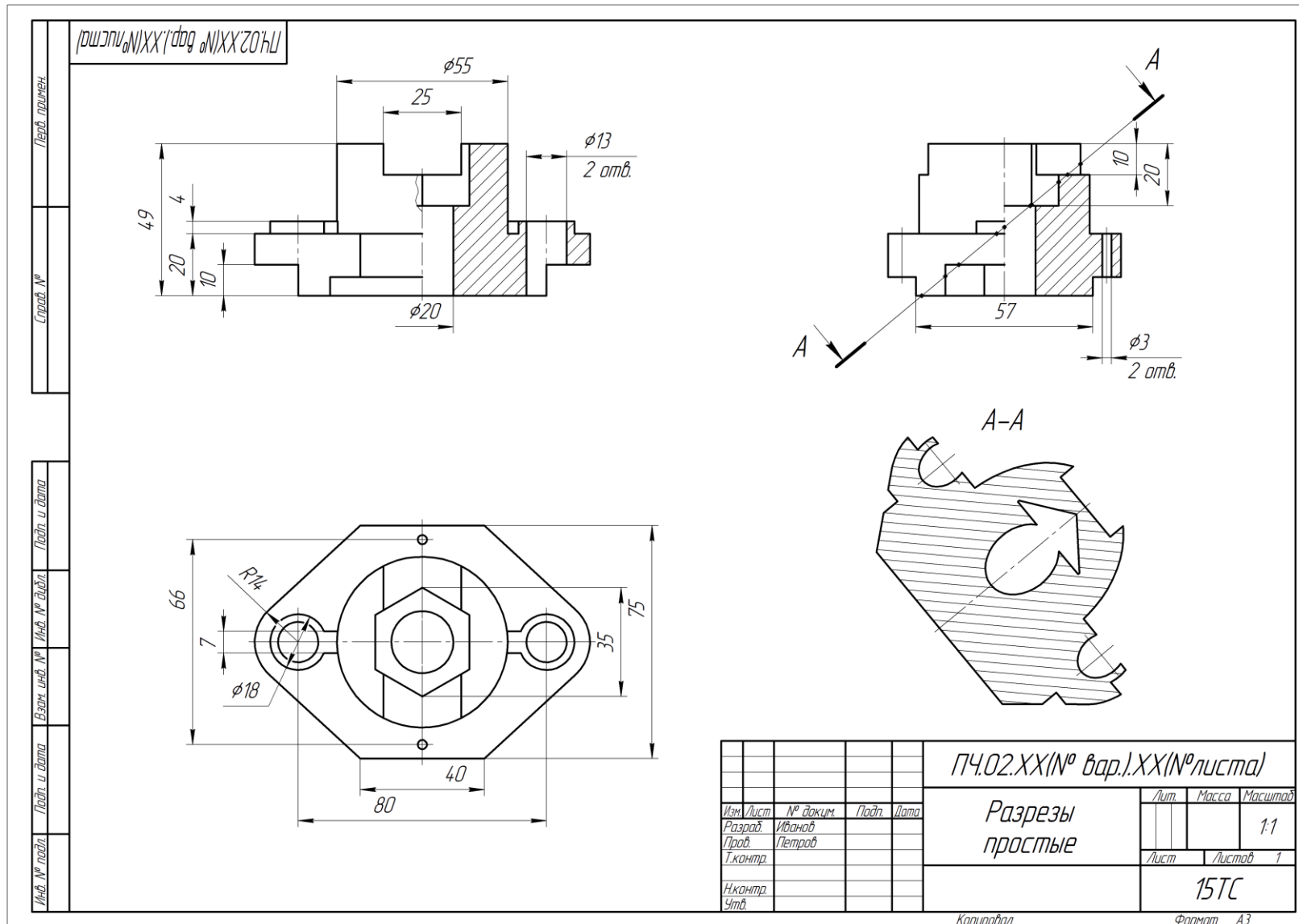
Рис. 9. Графическая работа по разделу «Инженерная графика». Тема «Проекционное черчение» (Лист 6 – Простые разрезы)
