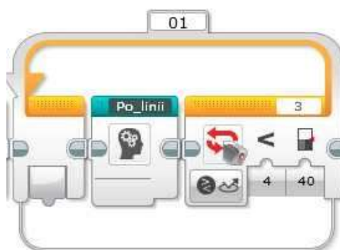
Рис.4. Алгоритм движения по линии до перекрёстка
