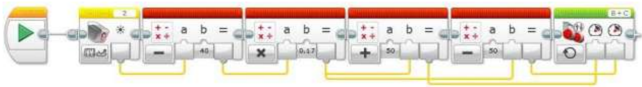
Рис.2. Алгоритм «по линии» на пропорциональном регуляторе
